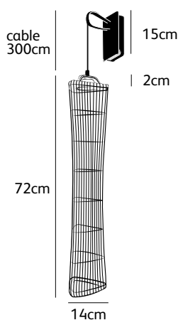
NP.07.WA.*
