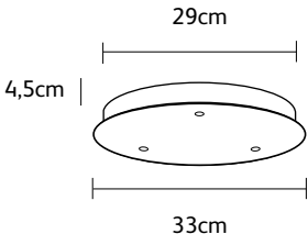
(c) NP.XL.DB.R.3L.*
