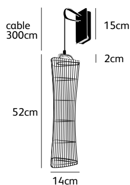
NP.05.WA.*
