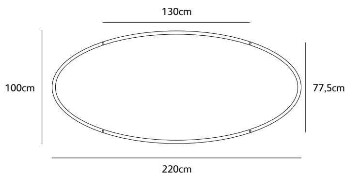
OV.220.SU.*
