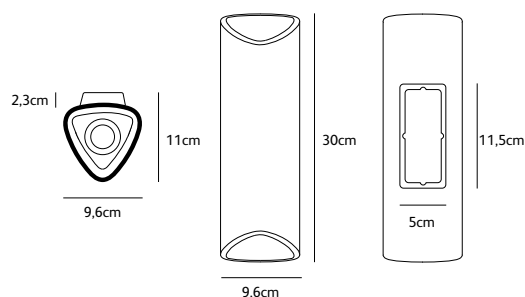
CK.OUTD.LED.BR
